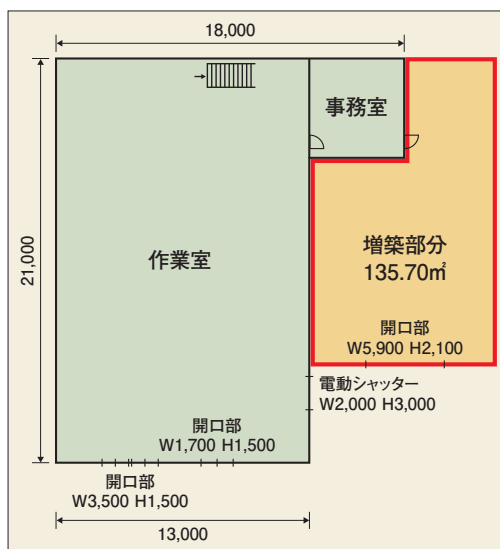
1階平面図(赤枠内が増築部分)
